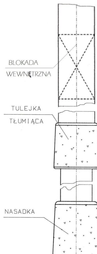
Rys.1 Regulacja bezstopniowa
